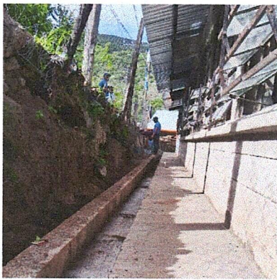
Foto 3: Cuneta de Concreto
